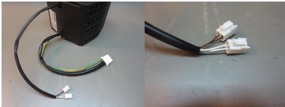
Εικόνα 4: Βοηθητικός Κινητήρας VF με Θερμικό Αισθητήρα χωρίς Encoder.
