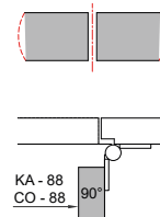
Λεπτομέρεια / Detail A
